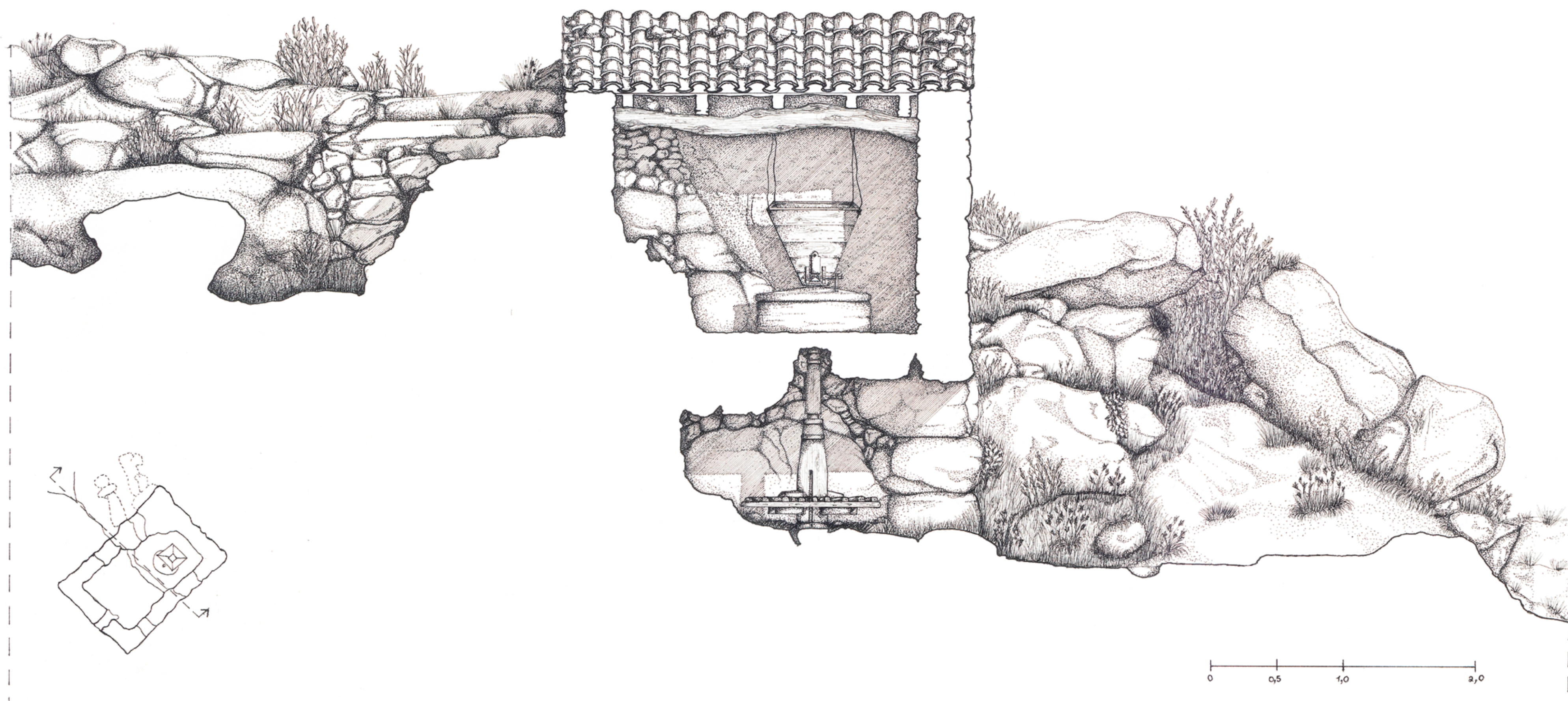
MOINHOS DO LAVADOURO, MEMBRA, MONTARIA, VIANA DO CASTELO. SEÇÃO LONGITUDINAL 1:25 10.10.2013 ANITA PIMENTA "LAVADOURO" WATERMILL, MONTARIA VIANA DO CASTELO CROSS SECTION 1:25 10.10.2013 ANITA PIMENTA
